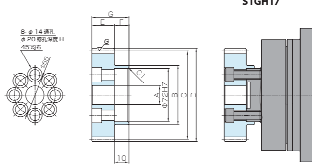
减速机型号 GH17 用小齿轮
