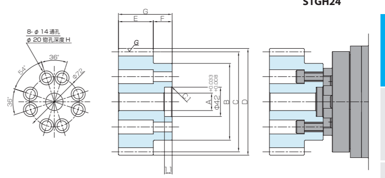
减速机型号 GH24 用小齿轮
